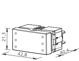
สวิตช์ ขนาด 1 ช่อง
