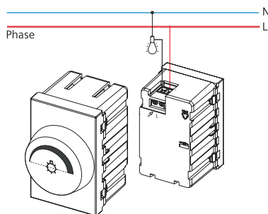
สวิตช์หรีฟ
