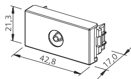
เต้ารับโทรทัศน์
