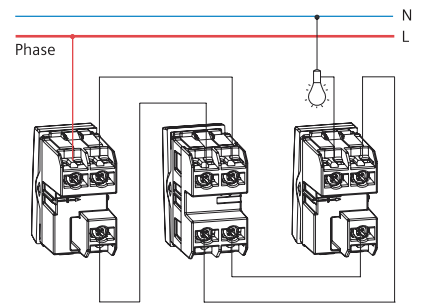
สวิตช์ 4 ทาง
